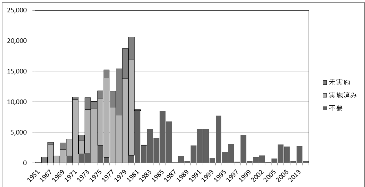
建物の建築年度別耐震改修工事の状況(床面積(m 2 )、年度)
