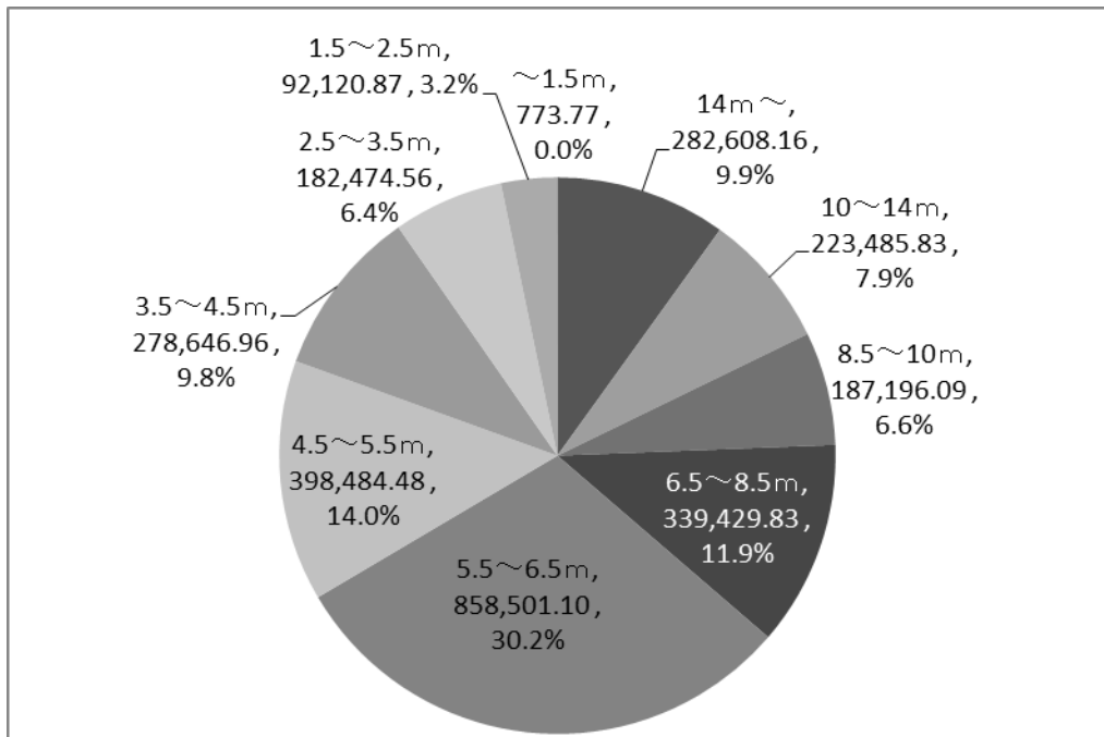
舗装道道路幅員別舗装面積(㎡) (～は以上・未満を示す)
